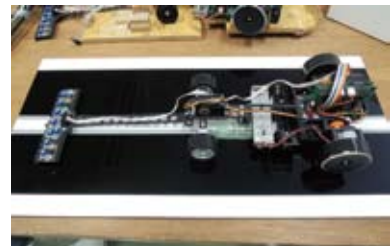
競技用マイコンカー
